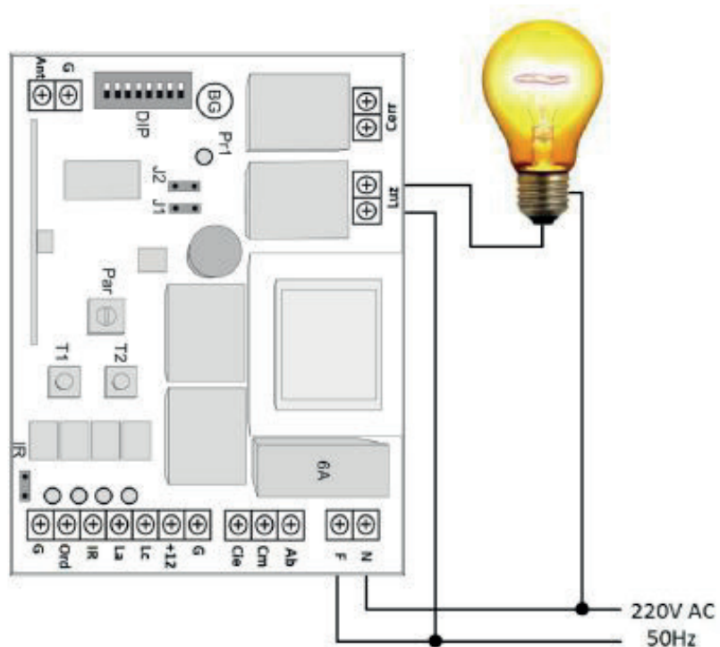
Esquema 3 - Conexión de Luz de Cortesia
