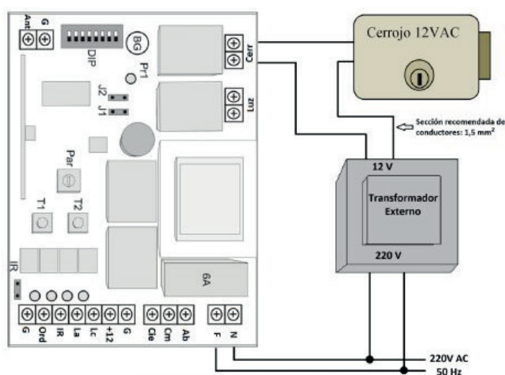
Esquema 1 - Conexión Electrocerradura 12V AC
