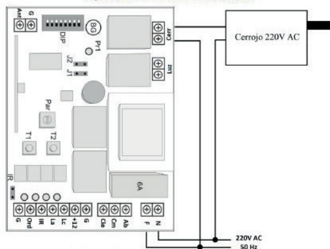
Esquema 2 - Conexión Electrocerradura 220V AC
