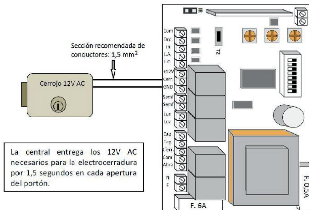
Esquema 1- Conexión de electrocerradura de 12V AC
