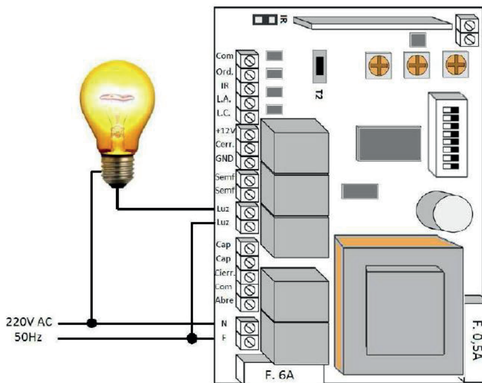
Esquema 2- Conexión de Luz de cortésia
