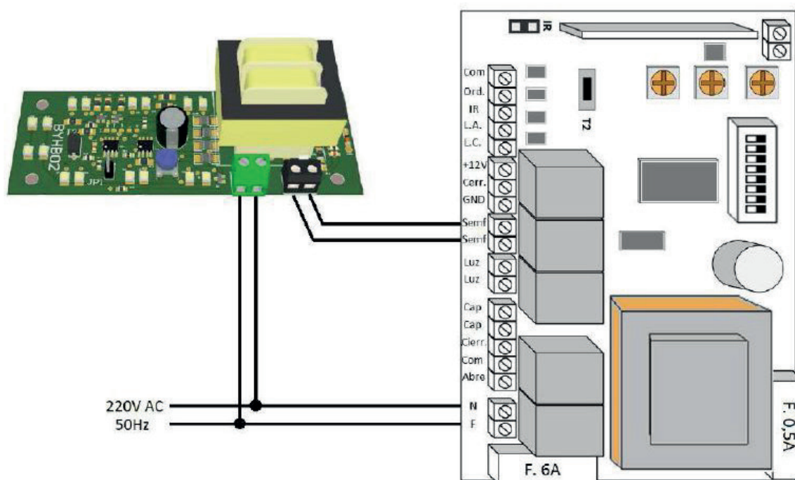
Esquema 4-Conexión de semáforo de 4 cables
