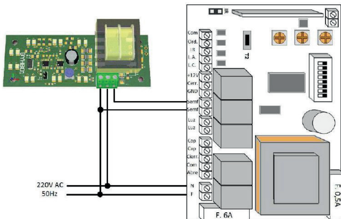
Esquema 3-Conexión de Semáforo de 3 cables
